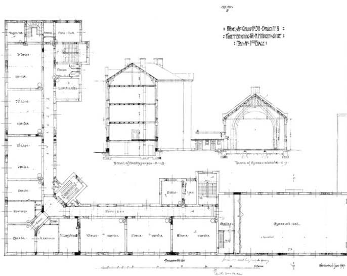
Plantegning for gymnastikkbygning, 1. etg. Opphavsrett: Statsbygg.
