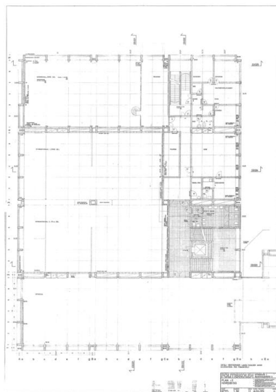
Plan 2. etasje. Foto: Arkitektene Lund og Slaatto. Opphavsrett: Statsbygg.
