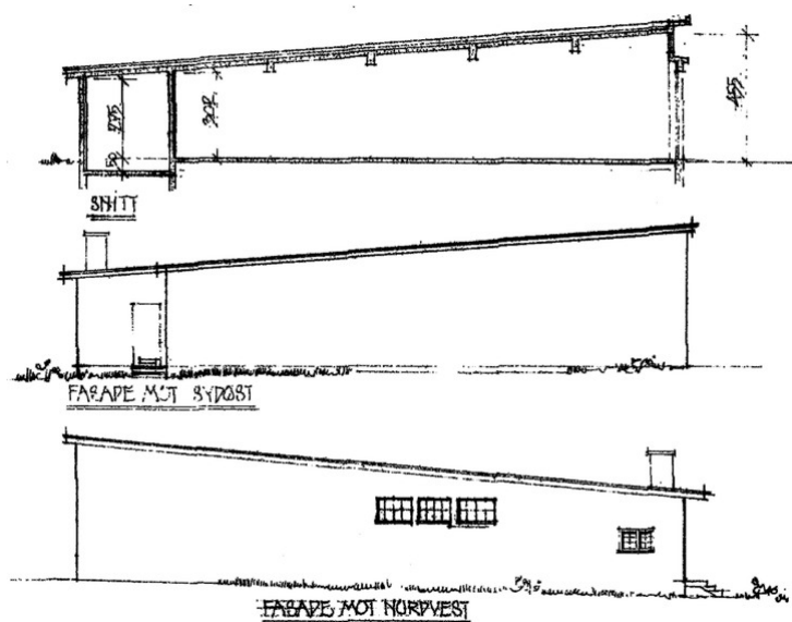
Snitt, samt fasader SØ og NV.
