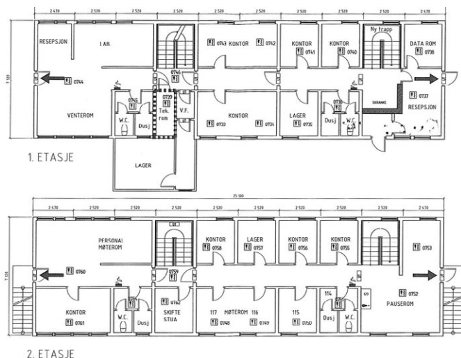
Plantegning 1. og 2. etasje.
