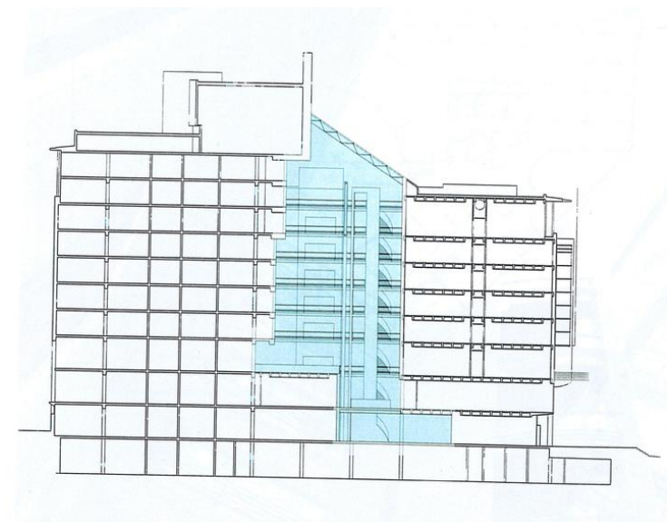
Snitt gjennom bygget Opphavsrett: Østgaard Arkitekter A/S.
