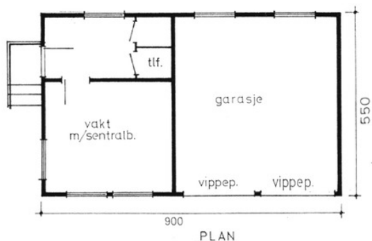
Plan- og snittegning.
