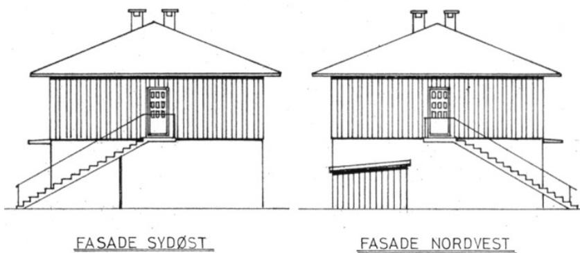
Endefasadene.
