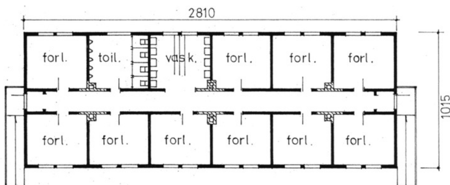
Plantegning 2. etasje, forlegningsrom.
