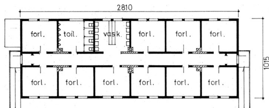
Plantegning 2. etasje, forlegningsrom.
