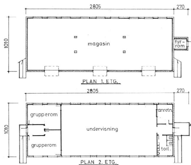
Plantegning 1. og 2. etasje.
