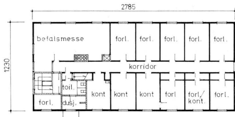
Plantegning 2. etasje med befalsmesse og -forlegning.
