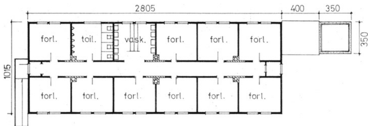
Plantegning 2. etasje.
