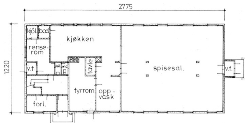
Plan 1. etasje med kjøkken og spisesal.
