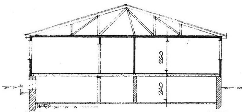
Snittegning.
