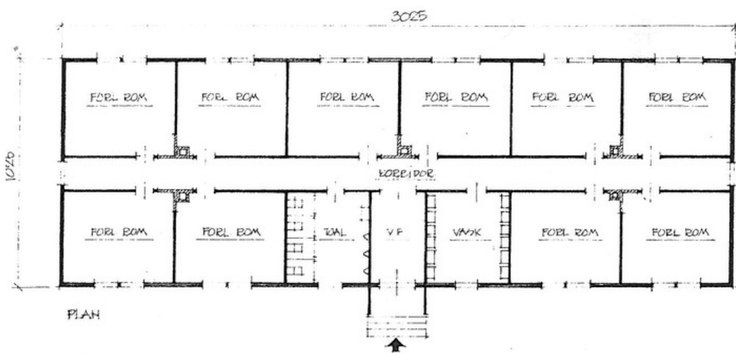
Plantegning 1. etasje. I dagens stand er flere av vinduene kledd igjen.
