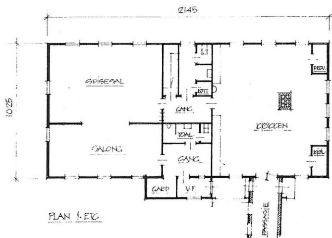
Plantegning 1. etasje.
