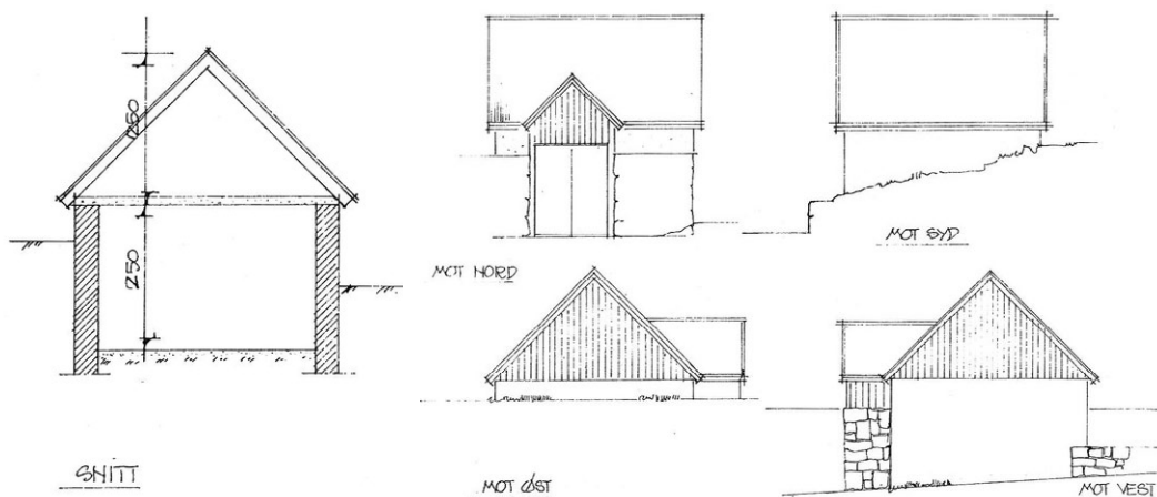
Fasadetegninger.
