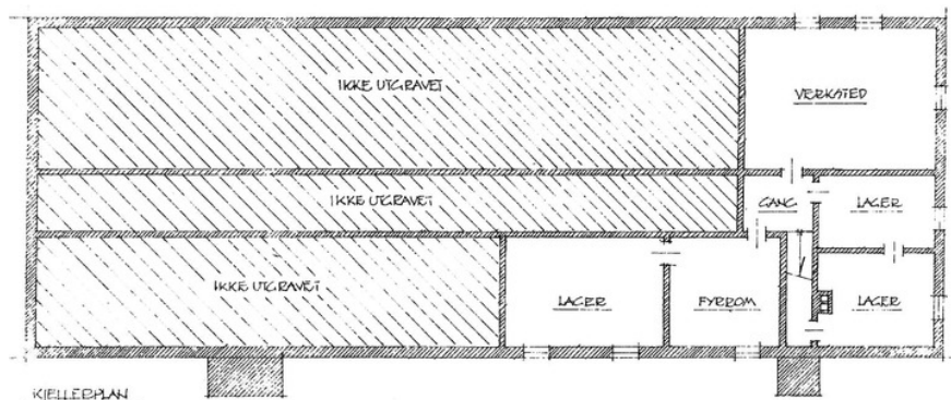
Plantegning kjeller.
