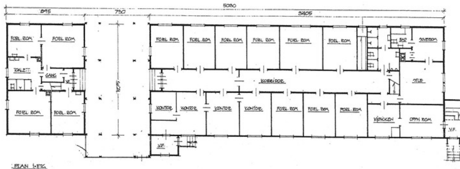
Plantegning 1. etasje.
