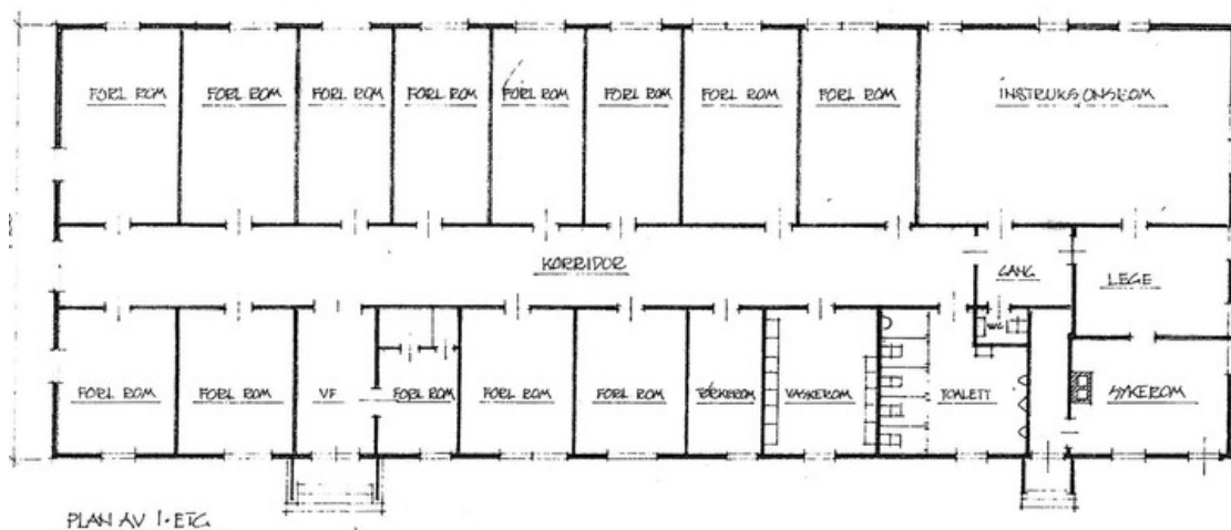
Plantegning 1. etasje.
