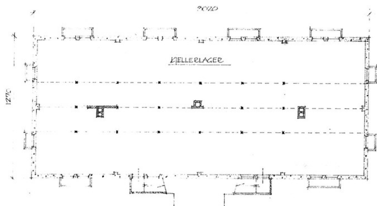
Plantegning kjeller.
