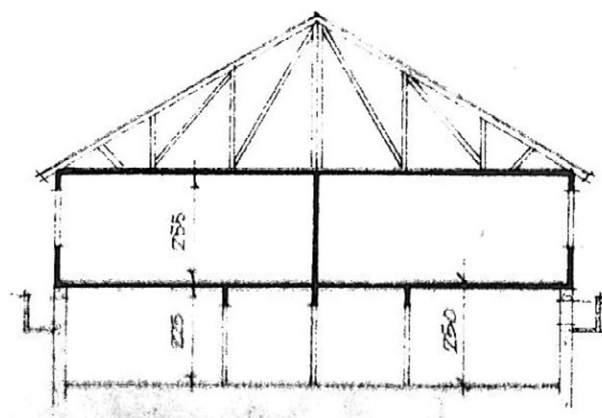
Snittegning.
