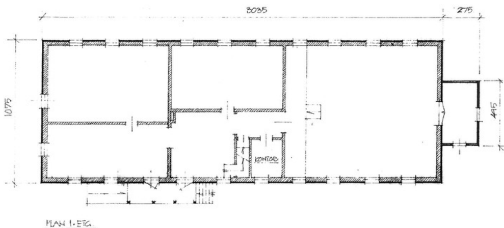
Plantegning 1. etasje.
