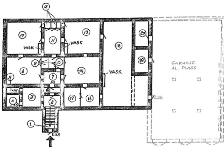
Plantegning for fjellanlegget.
