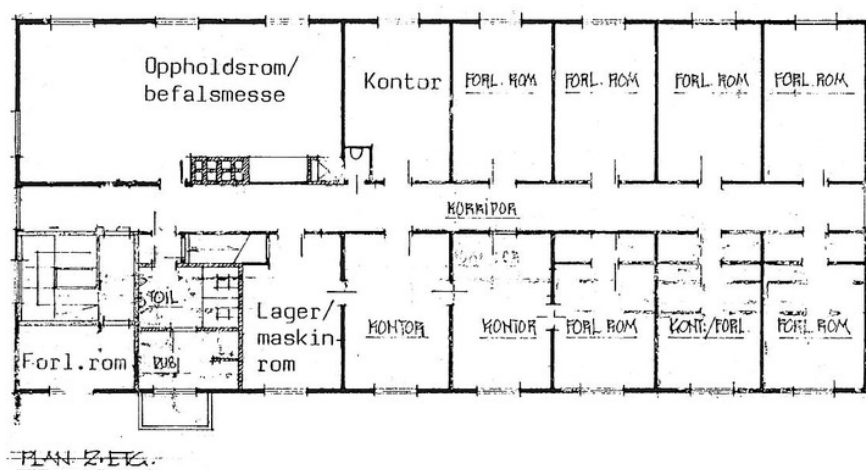
Plantegning 2. etasje.
