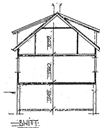
Snittegning.
