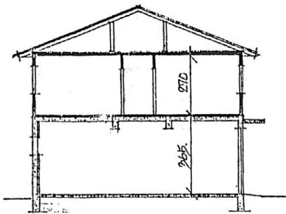
Snittegning.
