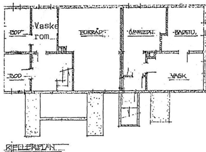
Plantegning kjelleretasje.
