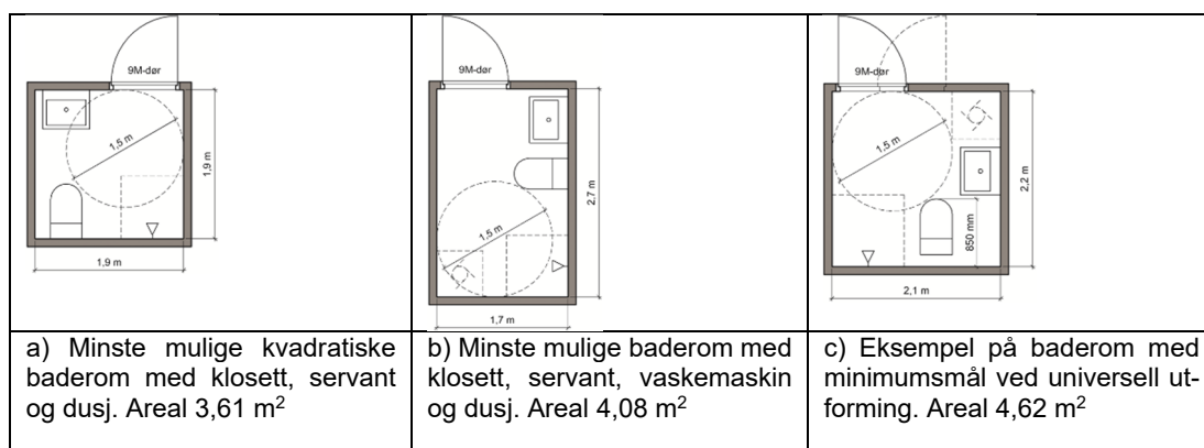
Figur 4.2. Eksempler på baderom med minimumsmål: a) og b) oppfyller TEK17, men ikke Husbankens kriterier for grunnlån, c) oppfyller Husbankens kriterier for grunnlån (Vegghengt klosettskål skal bygge minst 700 mm fra veggen, og mindre servant kan velges). Romdimensjoner i c) er i henhold til NS 11001-2:2018 og gjengitt i Byggforskeren 361.216.
