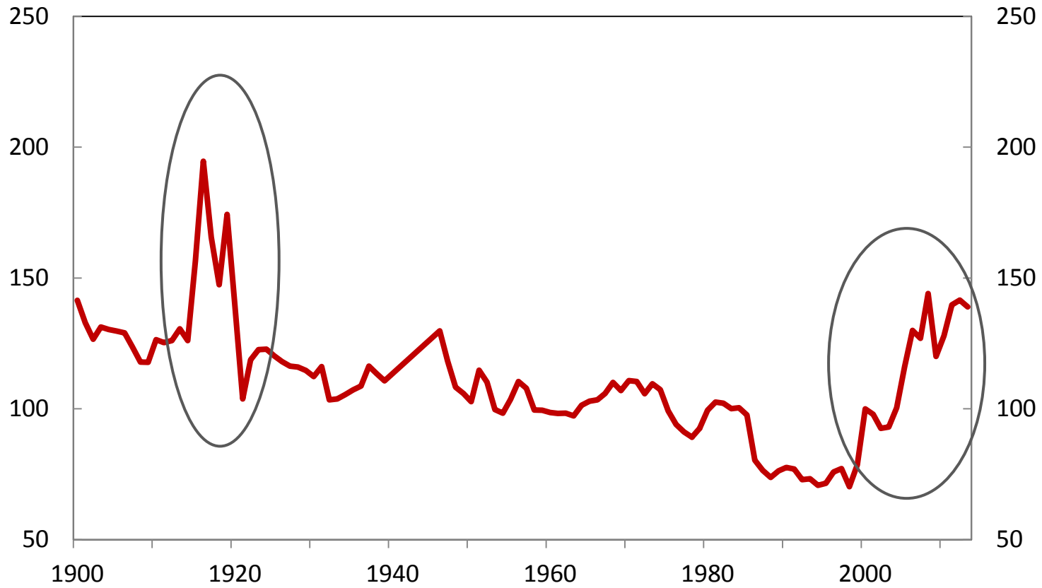
Bytteforhold 1990-2013. Indeks 2000=100
