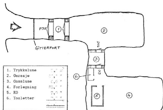
Alarmplassens plan med romangivelse.
