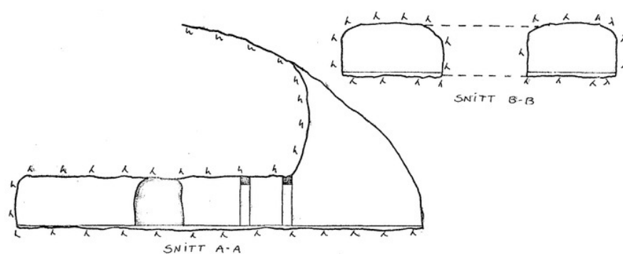
Snitt øst-vest og nord-sør.
