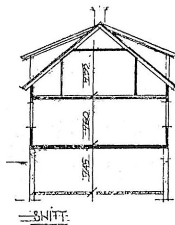
Snittegning.
