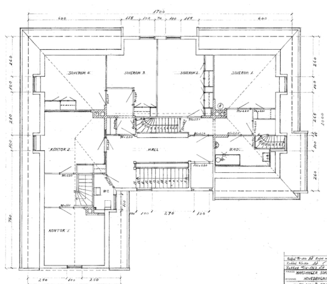
Plan av 2 etasje/loft. Opphavsrett: Statsbygg.
