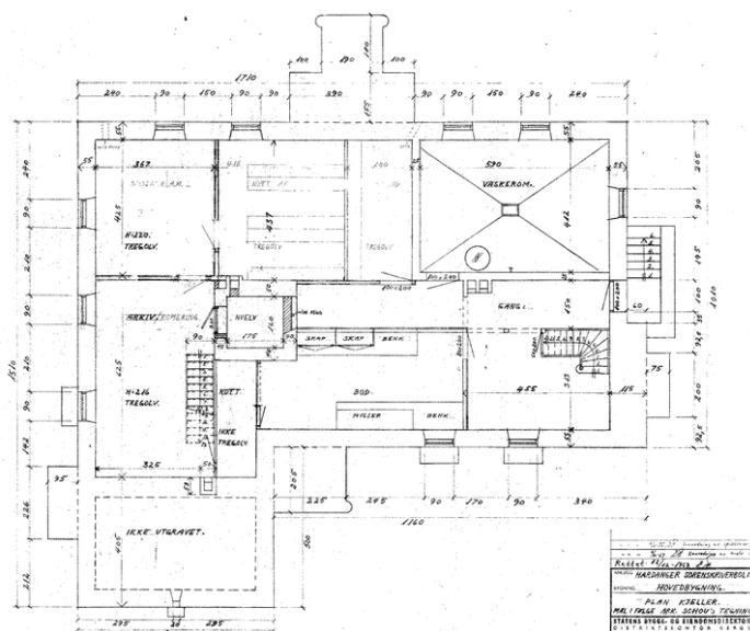
Kjellerplan. Opphavsrett: Statsbygg.
