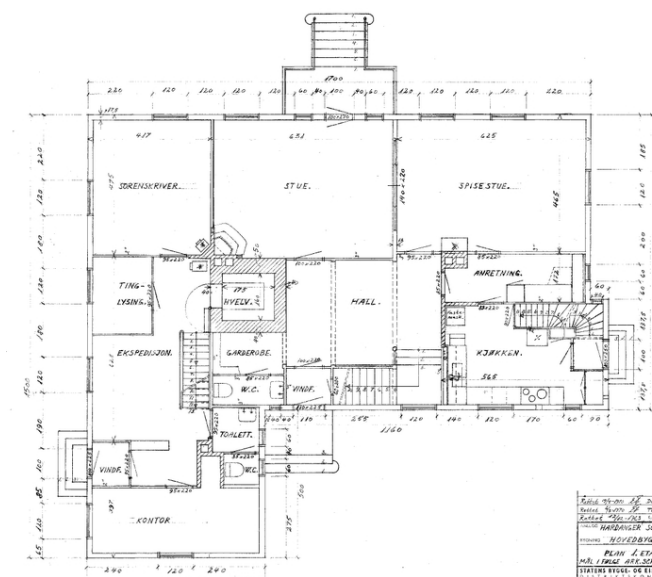
Plan av 1 etasje. Opphavsrett: Statsbygg.
