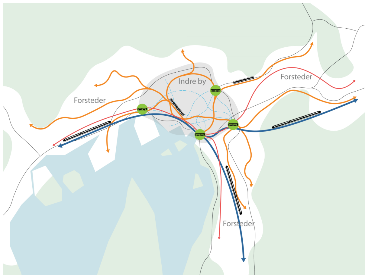
Figur 6-26: Prinsippskisse K4 Jernbane- og metrokonseptet.
