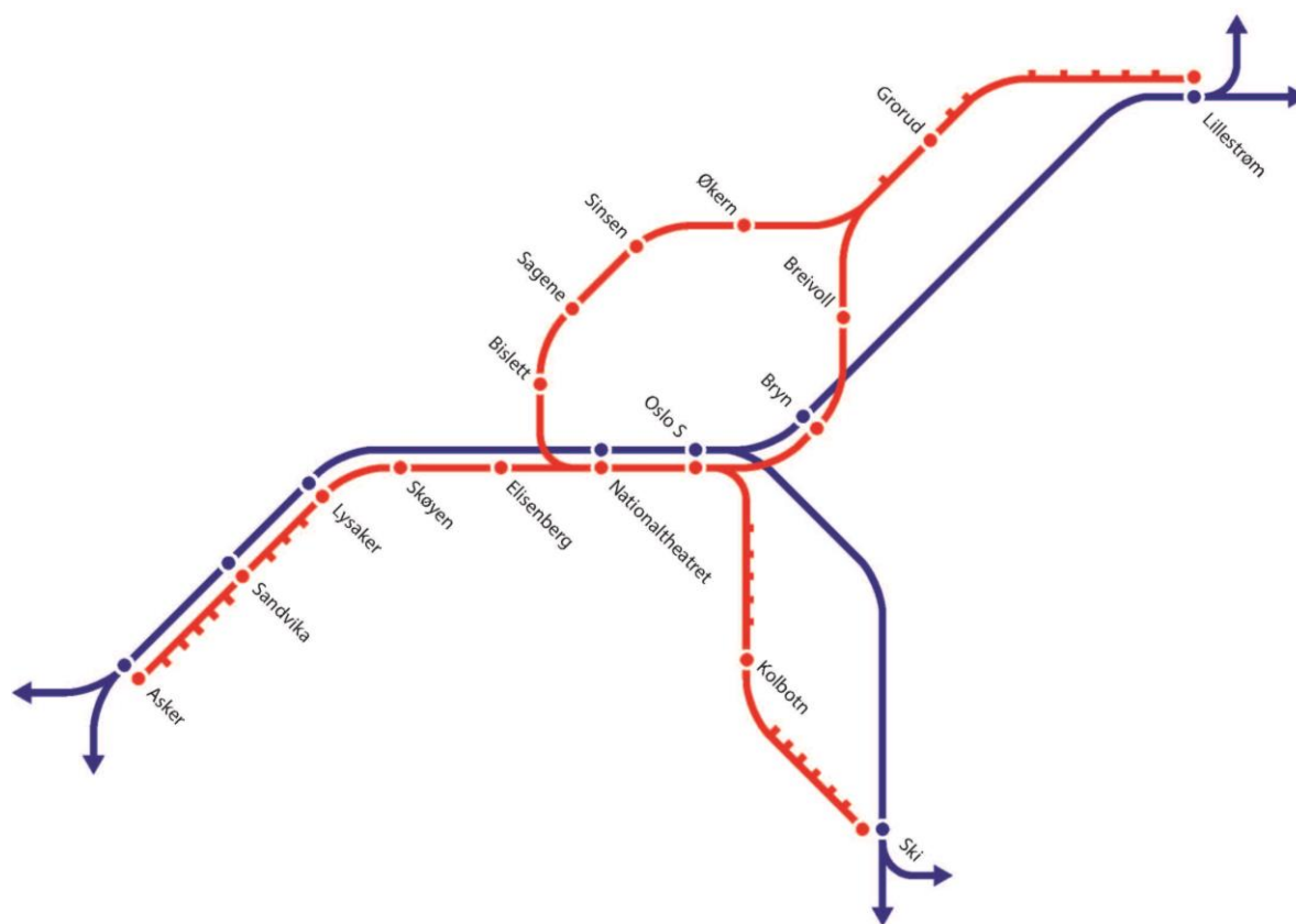
Figur 7-3 Prinsipper for separering av togtrafikken.
