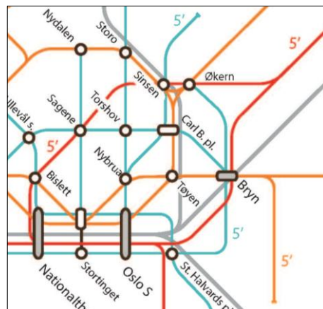
Figur 8-14 Linjenettet rundt Carl Berners plass.
