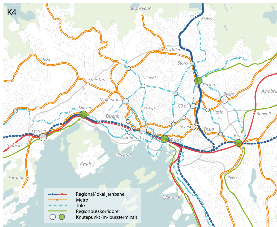
Figur 6-29: Geografisk nettnett- og knutepunktskart for skinnegående transport og regionbuss i K4
