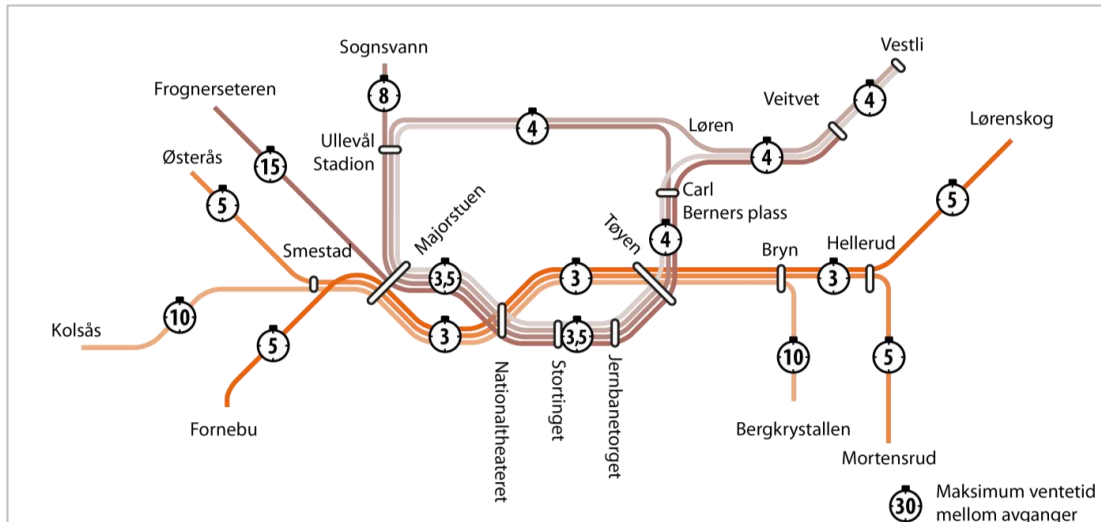
Figur 6-13: Overordnet tilbudskonsept for metro i K2. Største tid mellom avganger i minutter. Illustrasjonen viser det tilbudskonseptet som er beregnet i transportmodellen.
