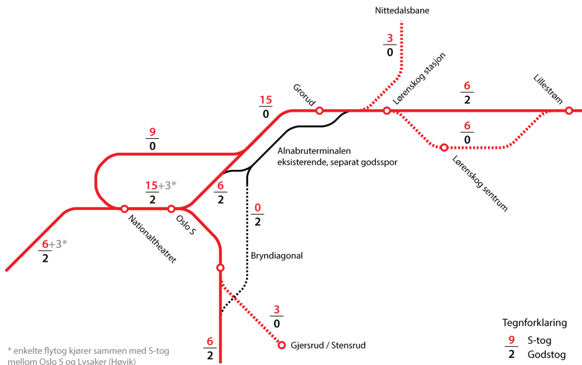
Figur 7-9 Stilisert utsnitt av S-banesystem i K3. Eksempel på tilbudskonsept som viser mulige utvidelser til grenbaner. Figuren viser antall tog i timen i en retning. (3* er tre tog Gardermoen–Stabekk i timen som kommer fra Romeriksporten).
