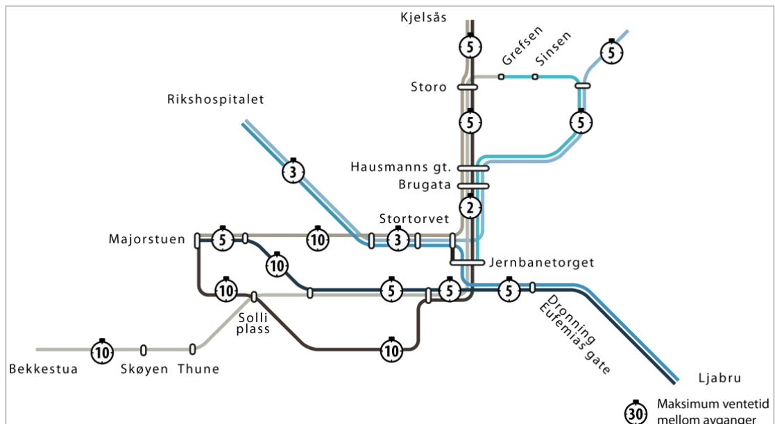
Figur 6-4 Overordnet tilbudskonsept for trikk i Nullalternativ+. Makstid mellom avganger i minutter. Illustrasjonen viser det tilbudskonseptet som er beregnet i transportmodellen.
