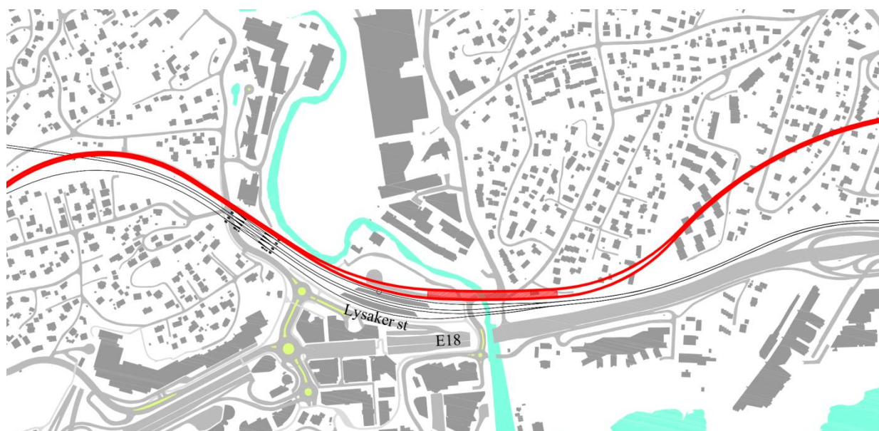
Figur 8-3: Utvidelse av Lysaker stasjon for lokaltog/S-bane.
