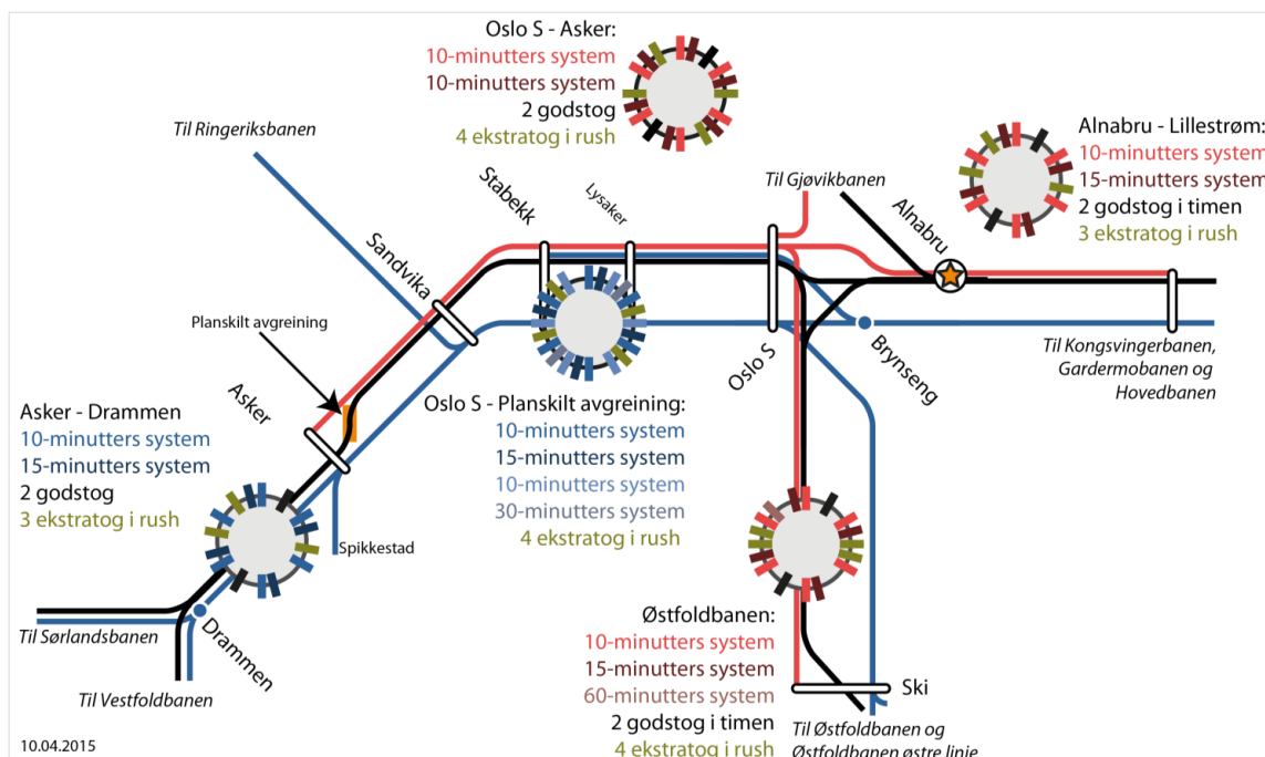
Figur 6-21 Godstog kjører sammen med S-bane og skifter over til regiontogsystem ved Hvalstad/ Billingstad. Eksempel på mulige taktkombinasjoner med to godstog i timen forutsatt infrastrukturiltak.
