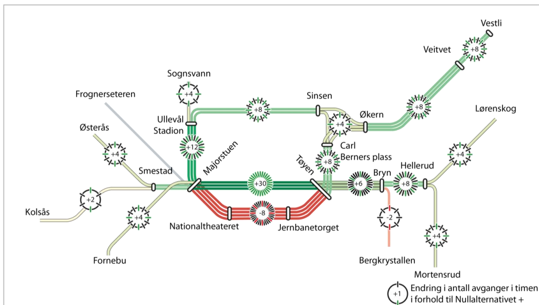
Figur 6-23 Metro i K3 – økt antall avganger pr. time sammenlignet med Nullalternativ+.
