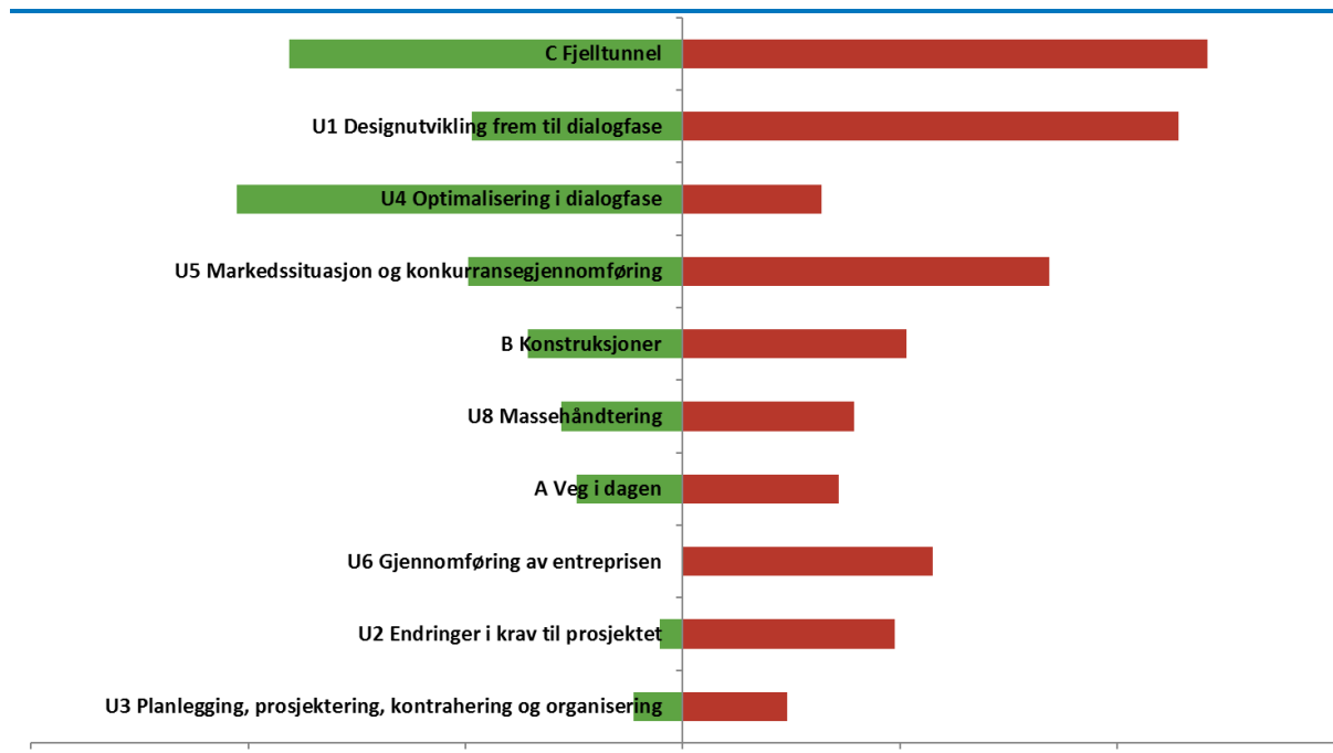
Figur 6-2: Bidrag til usikkerheten - Tornado
