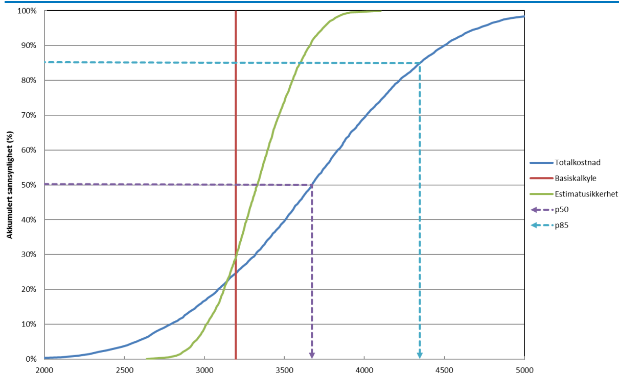
Figur 5-2 S-kurve inkl. mva., prisenivå 2018
