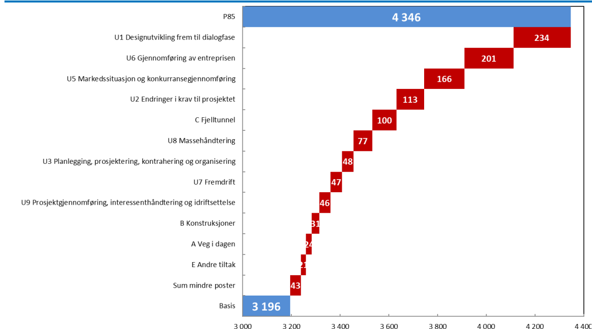
Figur 5-5 Bidrag til usikkerheten – fra basis til p85
