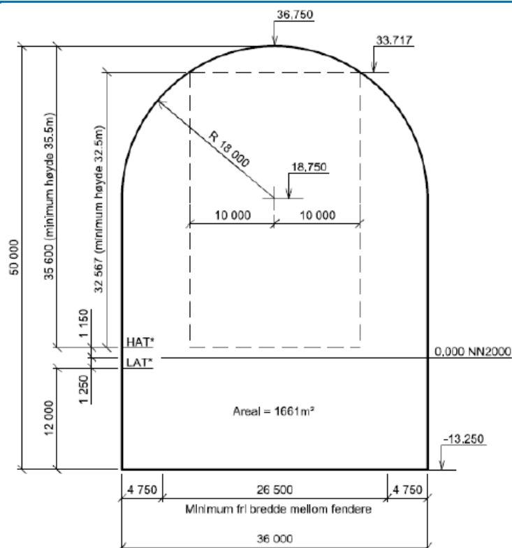
Figur 4-1: Planlagt tunneltversnitt. HAT: høyeste høyvann; LAT: Laveste lavvann
