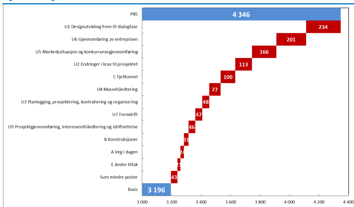
Figur 6-4 Bidrag til usikkerheten – fra basis til P85
